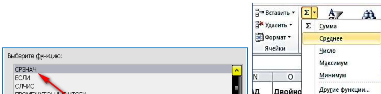
Рис. 22. Функция СРЗНАЧ
